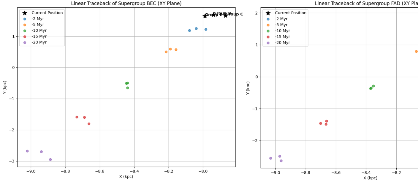
FIGURE 13 – Traceback linéaire des amas d'étoiles selon le plan galactique. À gauche : les amas B, E et C. À droite : les amas F, A et D. L'axe des abscisses représente la distance au centre galactique, et l'axe des ordonnées représente la tangente à la trajectoire de rotation moyenne de la galaxie au niveau du Cygne.
